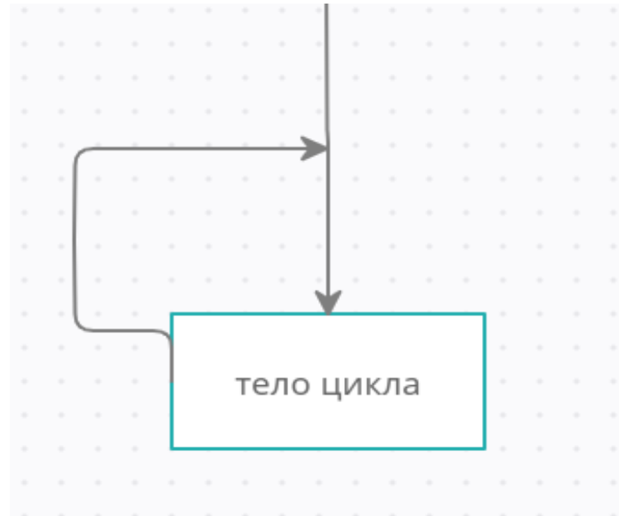
Рис. 126. Блок-схема цикла
