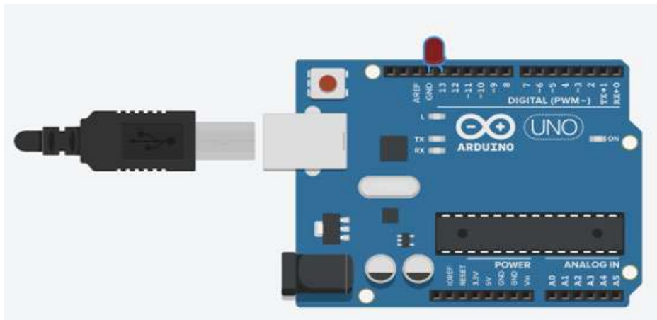
Рис. 165. Вид программы
