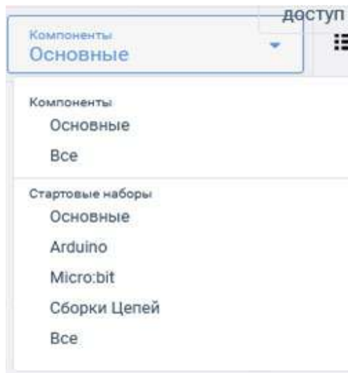
Рис. 168. Вид программы
