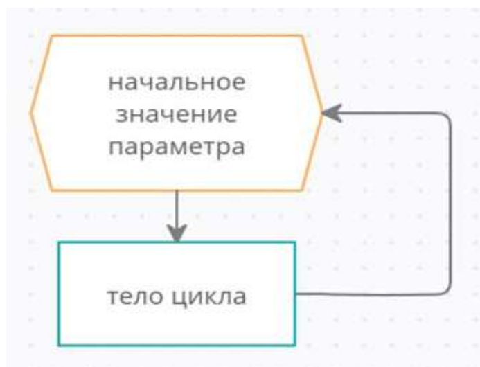
Рис. 124. Блок-схема цикла
