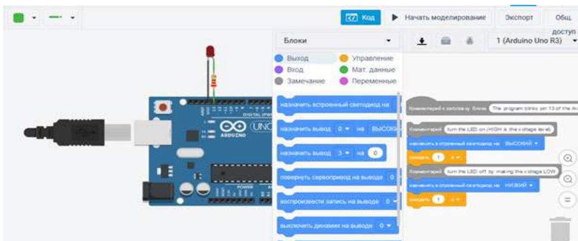
Рис. 171. Вид программы
