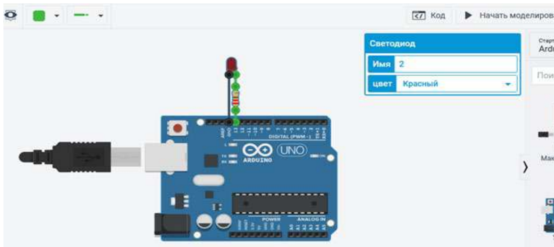
Рис. 170. Вид программы
