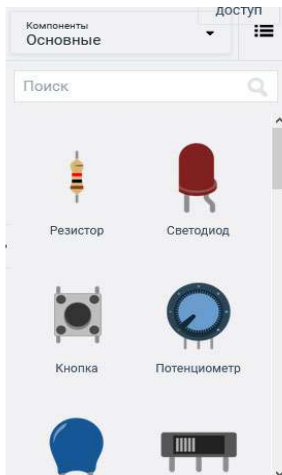
Рис. 167. Вид программы
