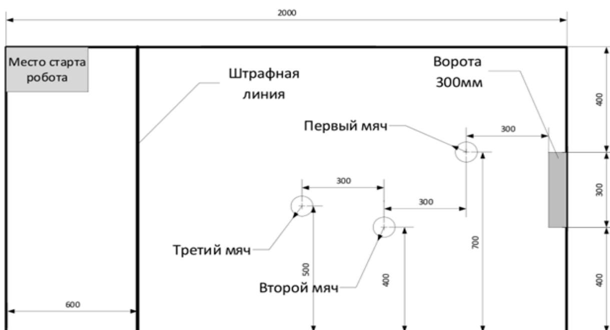
Рис. 179. Вид поля
