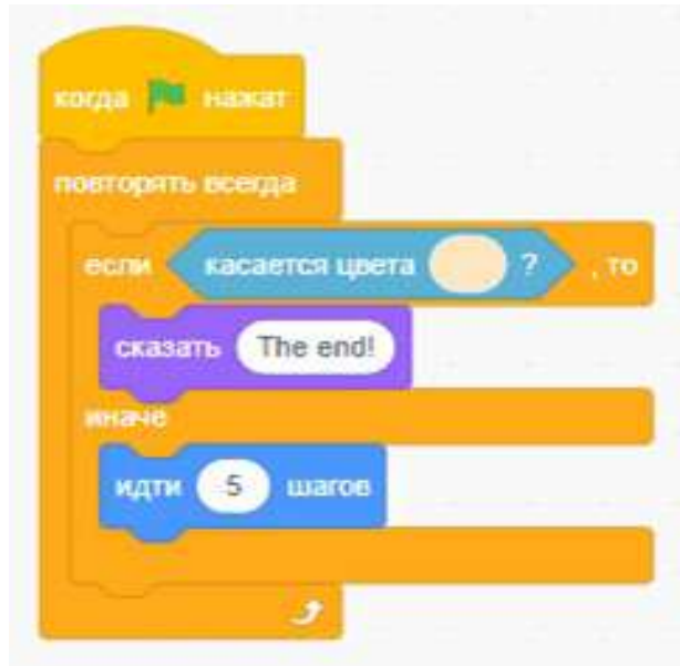
Рис. 129. Вид программы
